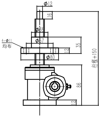
2A 螺母运动
